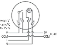
Fig 1b RTS114/ RTS114Q
